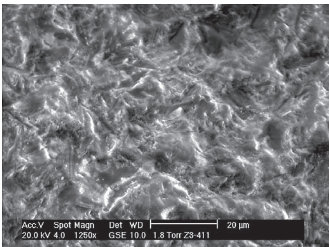
Abb. 2: Mikroskopische Aufnahme einer angerauten Zirkonoxidoberfläche/ Quelle: Zirkonoxidhersteller Metoxit AG
